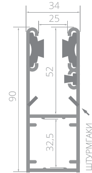
Профіль алюмінієвий екструдований *
