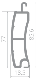
Профіль алюмінієвий екструдований *
